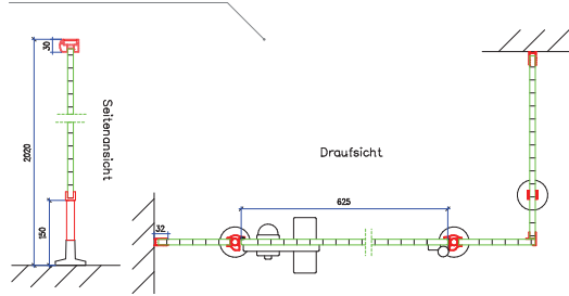
Schnittzeichnung
